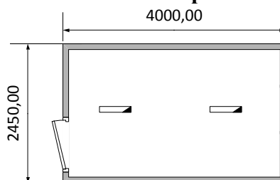
Схема планировки
